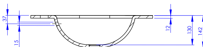
COUPE A-A
