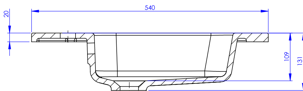
COUPE A-A
