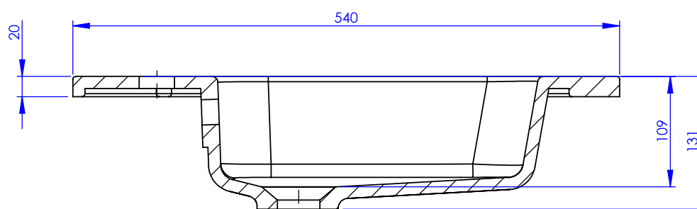
COUPE A-A
