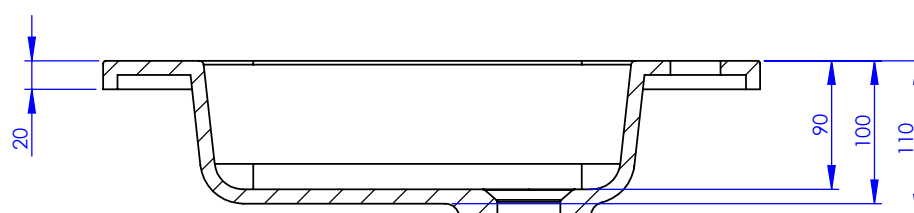
COUPE A-A
