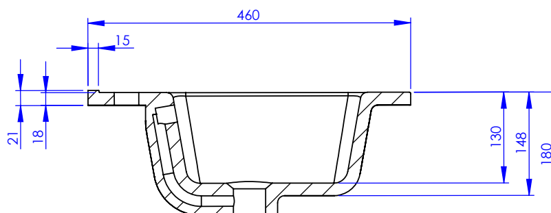
COUPE A-A
