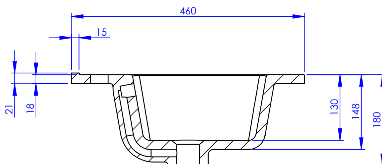
COUPE A-A
