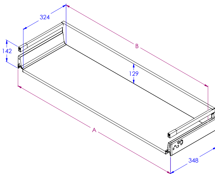
Casserolier - profondeur 460 mm
